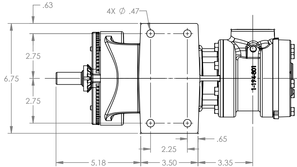
VIEW A-A
