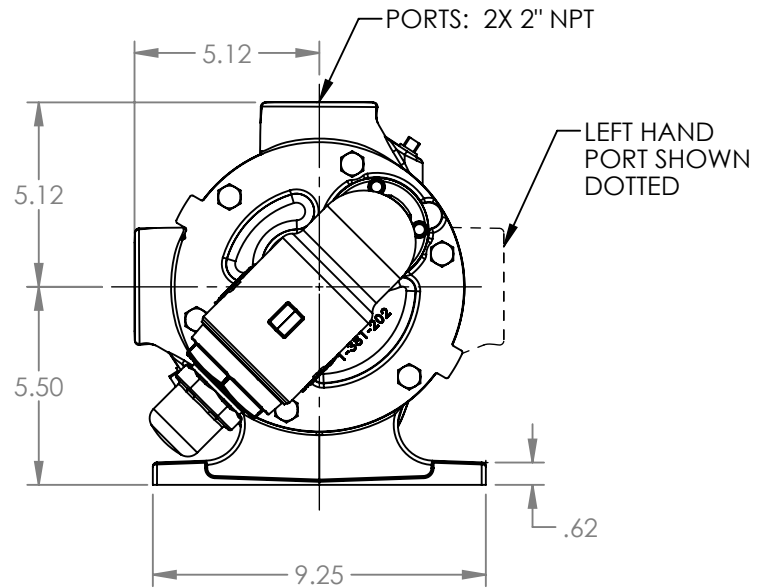
VIEW A-A
