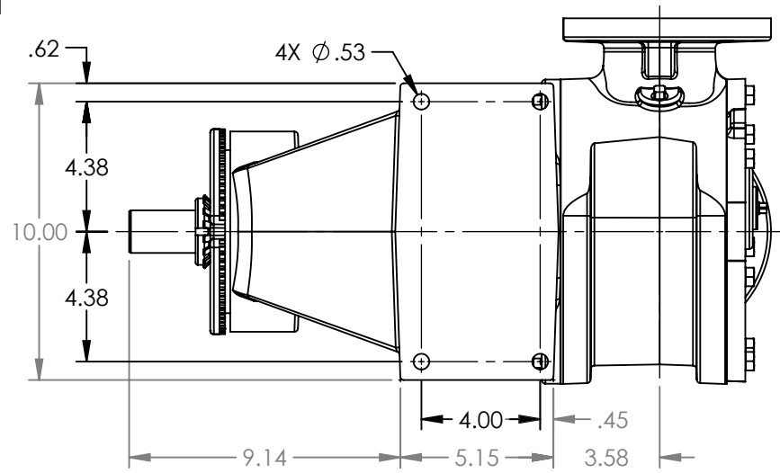
VIEW A-A
