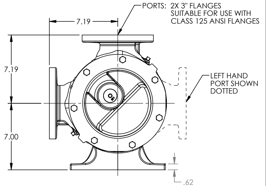
VIEW A-A
