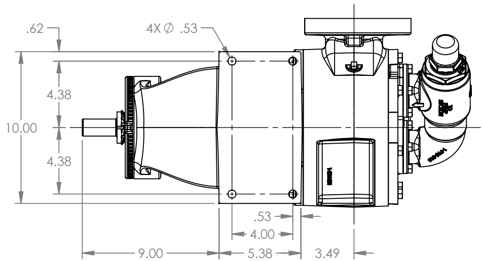
VIEW A-A
