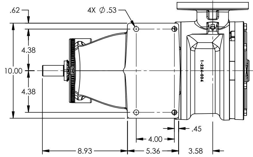
VIEW A-A
