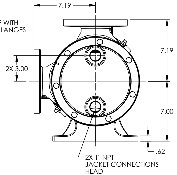
VIEW A-A
