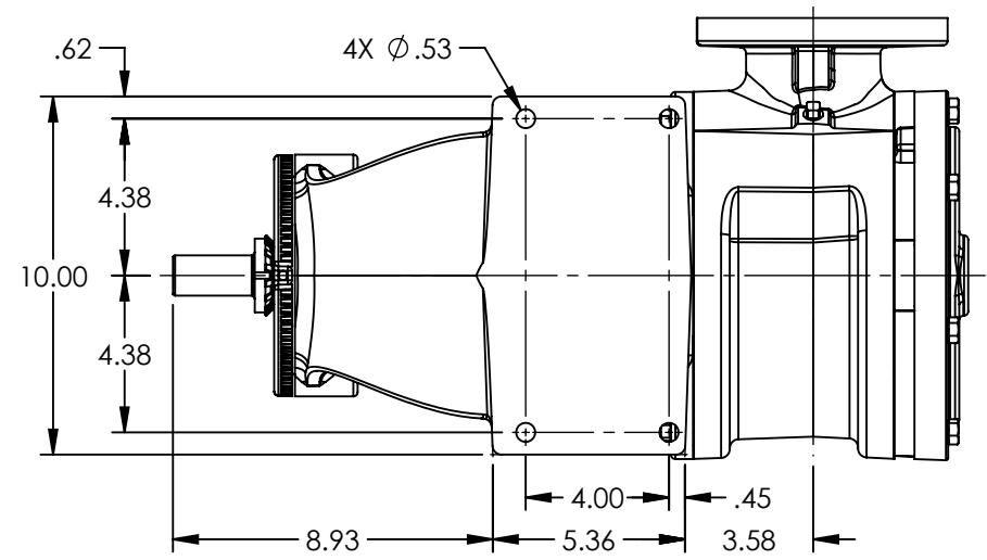
VIEW A-A
