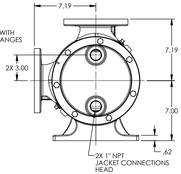
VIEW A-A
