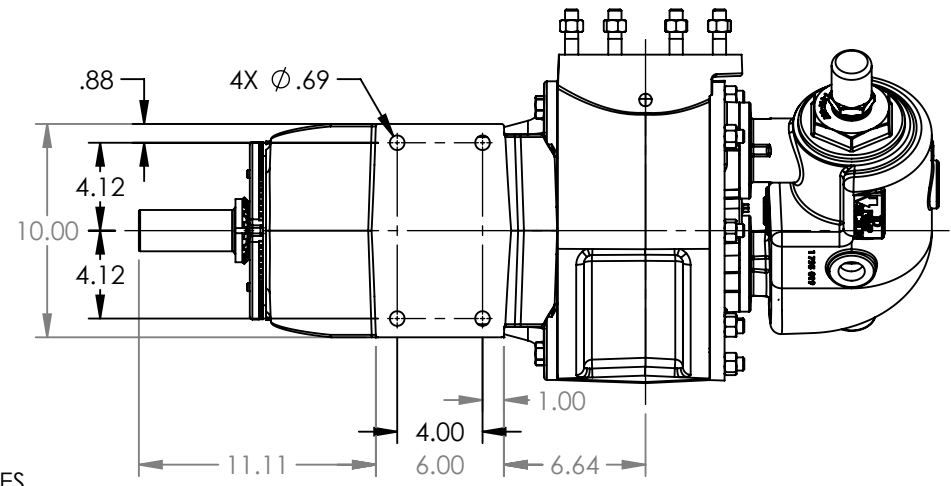
VIEW A-A
