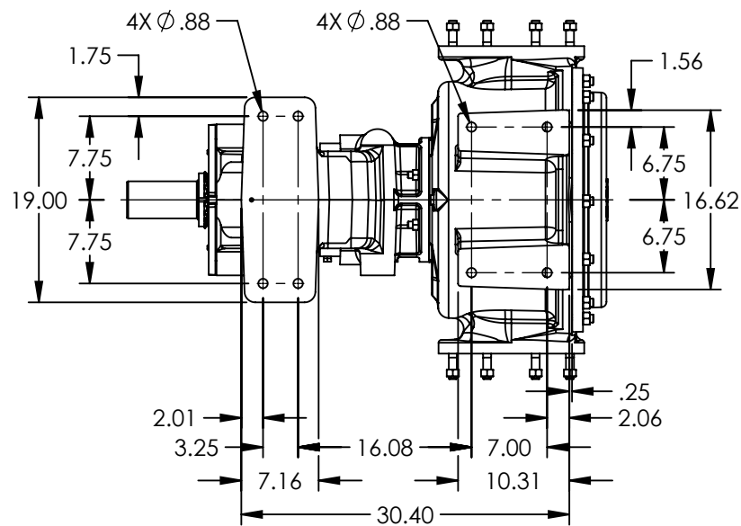
VIEW A-A
