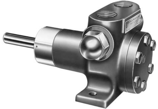
图 1 32 及 432 系列泵 (此处显示为 3 GPM 尺寸泵) 加填料或机械密封泵 阀门安装在泵体上 - 顺时针旋转
