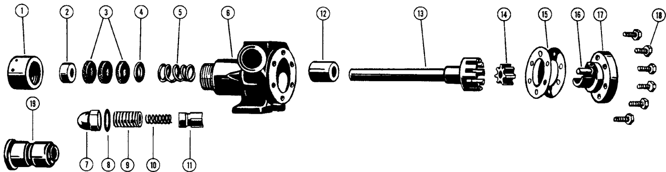
图 2 32 及 432 系列泵分解图
