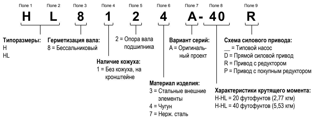
РИС. 3 СИСТЕМА ЧИСЛОВОЙ ИДЕНТИФИКАЦИИ МОДЕЛЕЙ ИЗДЕЛИЯ
