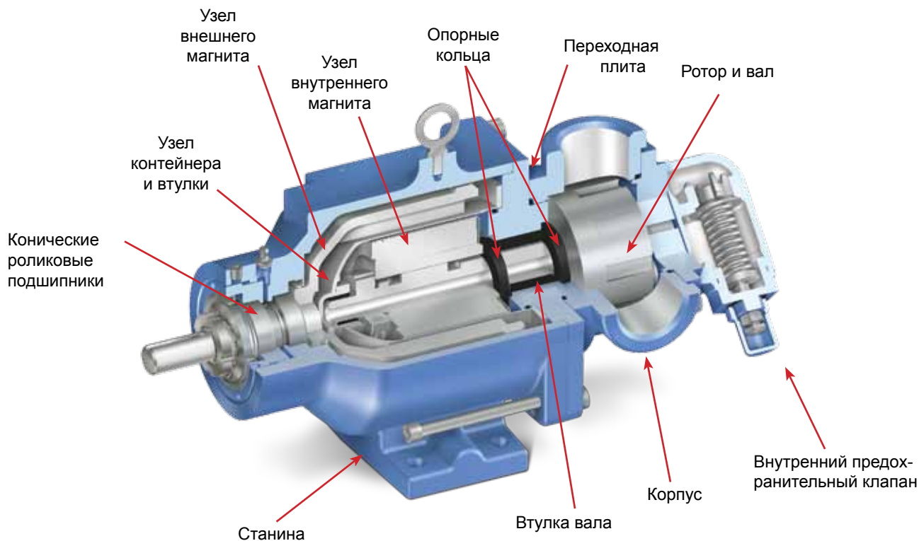
РИС. 4 ВИД В РАЗРЕЗЕ ТИПОВОГО НАСОСА С ЭЛЕКТРОМАГНИТНЫМ СИЛОВЫМ ПРИВОДОМ
