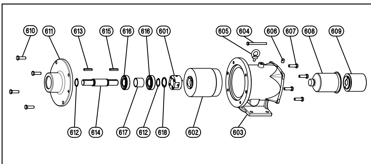
FIGURA 7 CONFIGURAZIONE TRASMISSIONE M MD2 – COMPONENTI PORTANTE DEI CUSCINETTI E ACCOPPIAMENTO SERIE B
