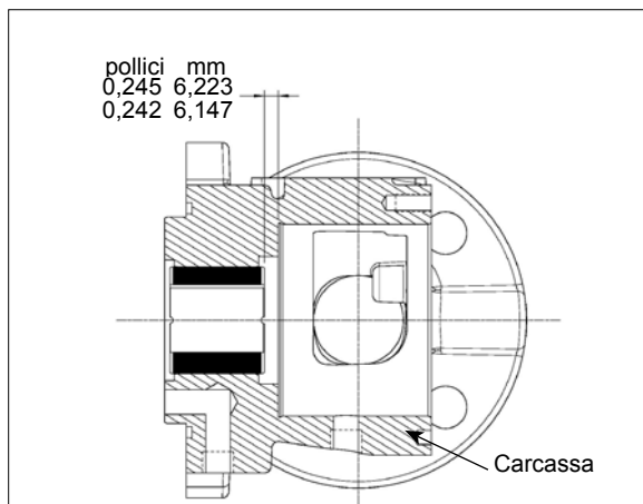
FIGURA 15 POSIZIONAMENTO DELLA BOCCOLA DELLA CARCASSA
