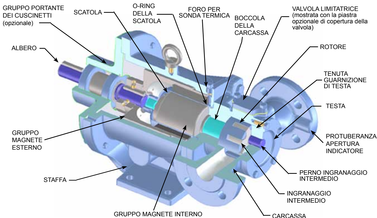
FIGURA 4 ILLUSTRAZIONE DELLA SEZIONE TRASVERSALE DELLA POMPA MAG DRIVE MD2-B CON PORTANTE DEI CUSCINETTI
