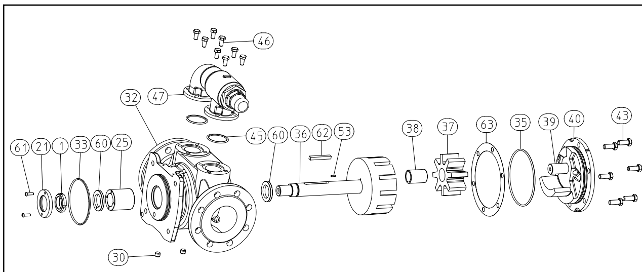
FIGURA 6 RAPPRESENTAZIONE ESPLOSA – POMPE MAG DRIVE MISURA AS, AK, AL, KE E KKE
