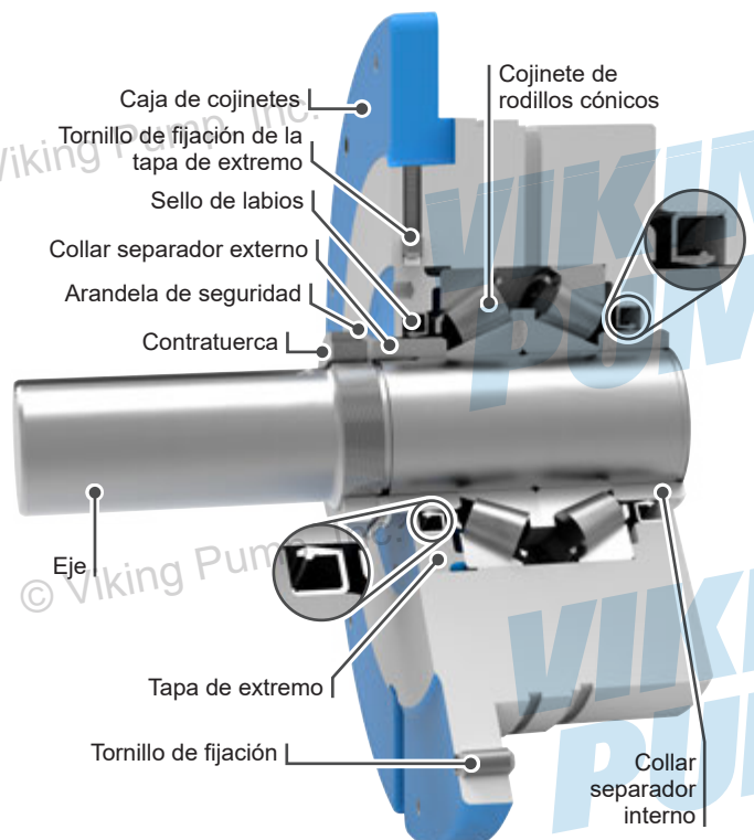
FIGURA 7: CONJUNTO DE CAJA DE COJINETES
