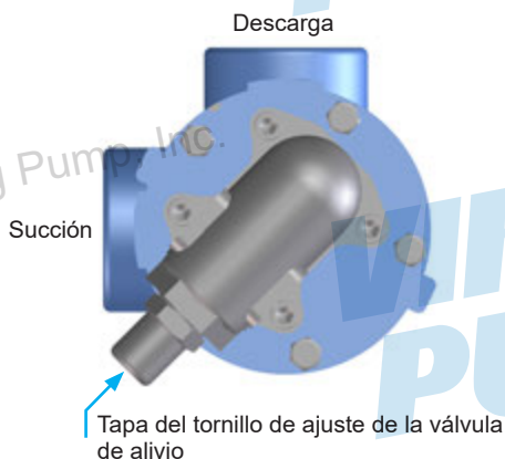
FIGURA 3: POSICIÓN DE LA VÁLVULA DE ALIVIO
