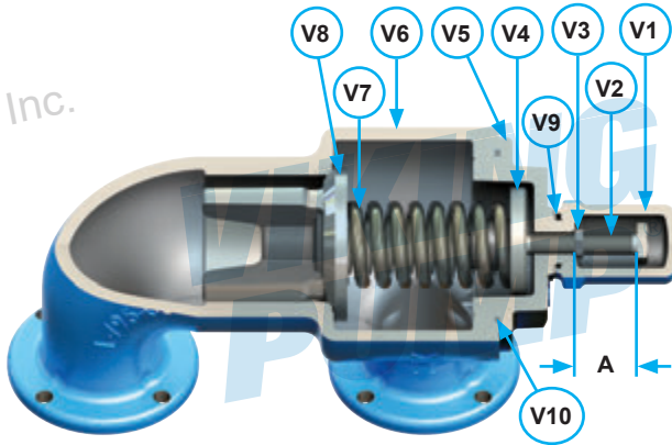
FIGURA 9: VÁLVULA DE ALIVIO: TODOS LOS TAMAÑOS NOTA: La imagen es solo representativa.
