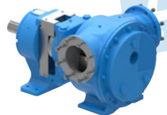
FIGURA 2: TAMAÑOS N, R, RS
