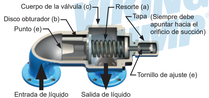
FIGURA A5-A: VÁLVULA DE ALIVIO DE PRESIÓN INTERNA
