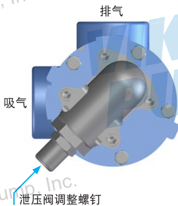
图 5：泄压阀位置
