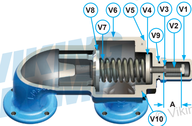
阀 - 零件列表
