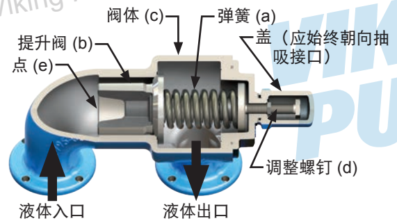
图 A4: 威肯内部 泄压阀的剖视图
