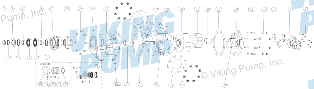
图 8: 分解图 (Q、QS 尺寸) — 124A SERIES™、4124A SERIES™、224A SERIES™、4224A SERIES™ 注: 图像仅具有代表性
