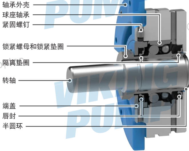
图 16: 轴承外壳组件 (K、KK、LQ、LL、LS)
