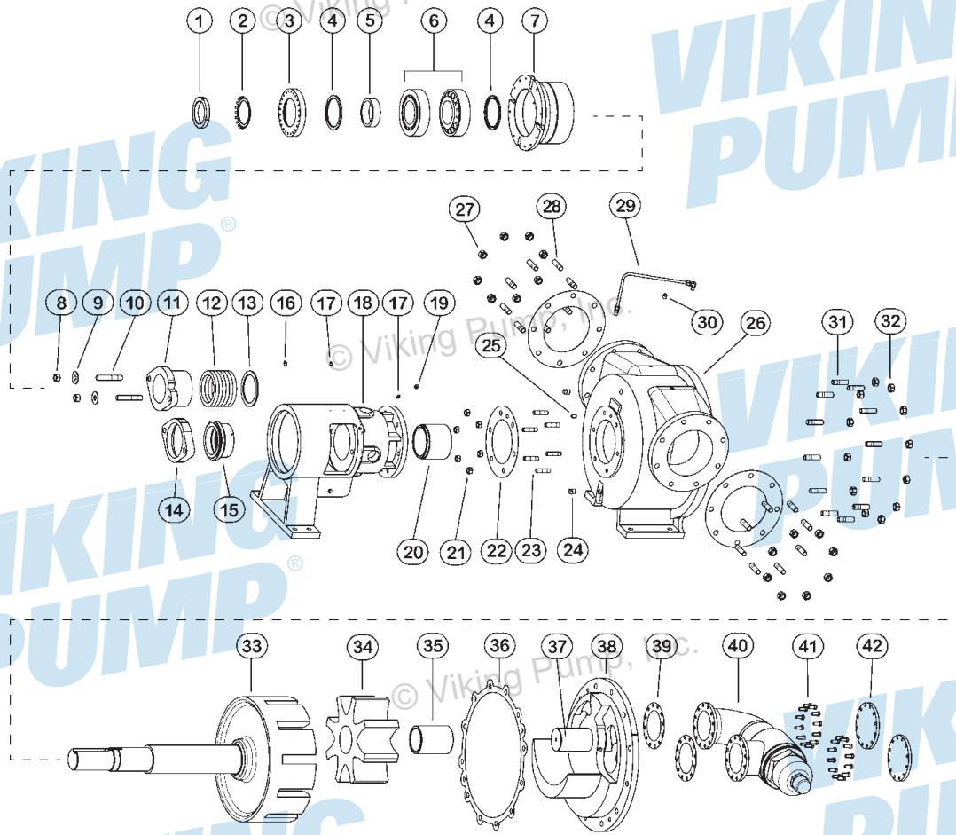
图 9：分解图（N、R、RS 尺寸）— 324A SERIES™、4324A SERIES™
