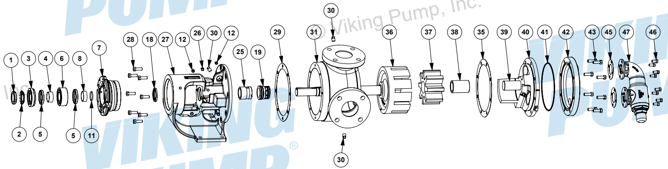
图 7: 分解图 (G、H、HL、AK、AL、K、KK、L、LQ、LL、LS 尺寸) — 4124B SERIES™、4224B SERIES™ 注: 图像仅具有代表性
