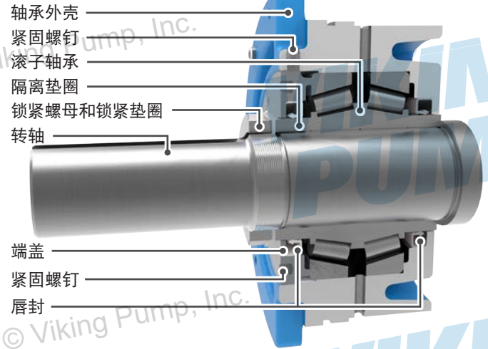
图 17: 轴承外壳组件 (Q、QS、N、R、RS)
