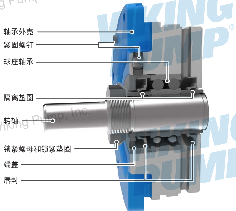
图 15: 轴承外壳组件 (H、HL)
