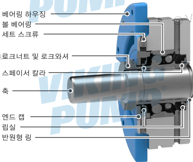
그림 10: 베어링 하우징 조립체 (K, KK, L, LQ, LL, LS)
