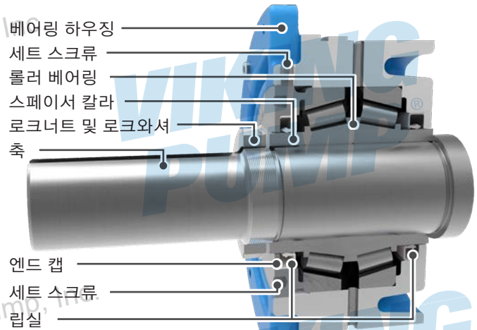
그림 11: 베어링 하우징 조립체 (Q, QS)
