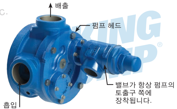
그림 A5-B: RTR(RETURN TO TANK) 압력 배출 밸브
