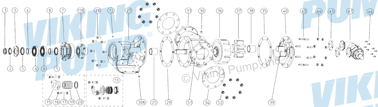
그림 5: 분해도(Q, QS 크기) — 126A SERIES™, 4126A SERIES™, 226A SERIES™, 4226A SERIES™ 주의사항: 참조용 이미지입니다.
