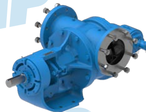
그림 3: Q, QS 크기 (QS126A 표시)
