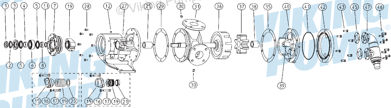
그림 4: 분해도(H, HL, K, KK, L, LQ, LL, LS 크기) — 126A SERIES™, 4126A SERIES™, 226A SERIES™, 4226A SERIES™ 주의사항: 참조용 이미지입니다.
