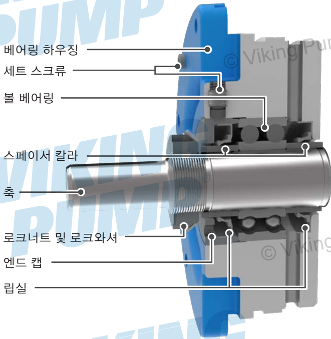
그림 9: 베어링 하우징 조립체(H, HL)
