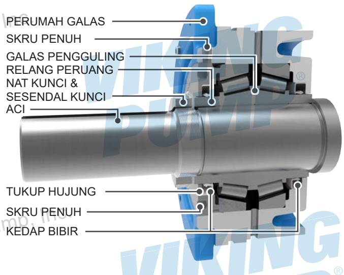
RAJAH 11: PEMASANGAN PERUMAH GALAS (Q, RS)
