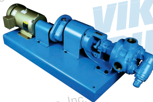
RAJAH A12: PEMACUAN PENGECIL
