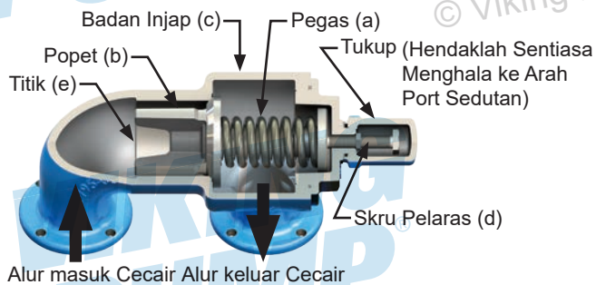
RAJAH A5-A: INJAP PELEGA TEKANAN DALAM
