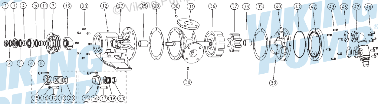
RAJAH 4: PANDANGAN TERBURAI (SAIZ H, HL, K, KK, L, LQ, LL, LS) — 126A SERIES™, 4126A SERIES™, 226A SERIES™, 4226A SERIES™ NOTA: IMEJ ADALAH WAKIL SAHAJA
