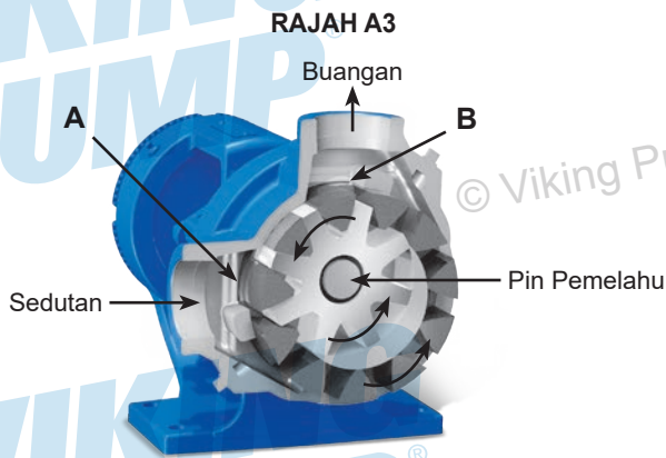
RAJAH A4: PEMUTUSAN DALAM VIKING INJAP PELEGA TEKANAN
