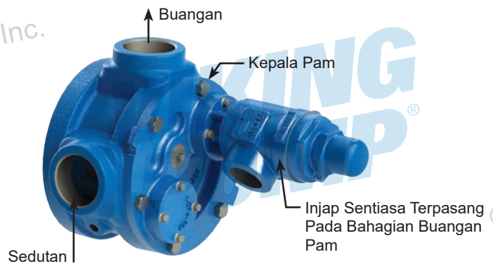
RAJAH A5-B: INJAP PELEGA TEKANAN KEMBALI KE TANGKI
