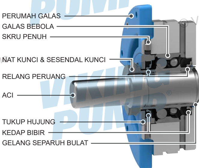
RAJAH 10: PEMASANGAN PERUMAH GALAS (K, KK, L, LQ, LL, LS)
