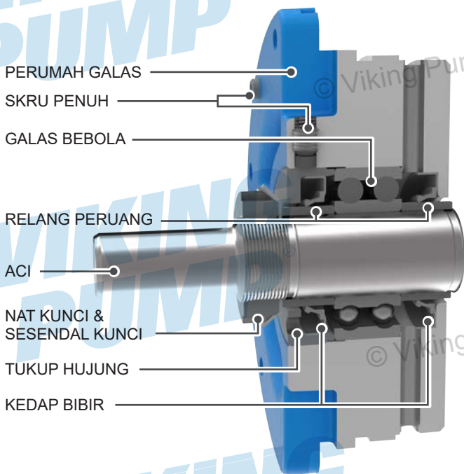
RAJAH 9: PEMASANGAN PERUMAH GALAS (H, HL)
