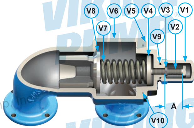
阀 - 零件列表
