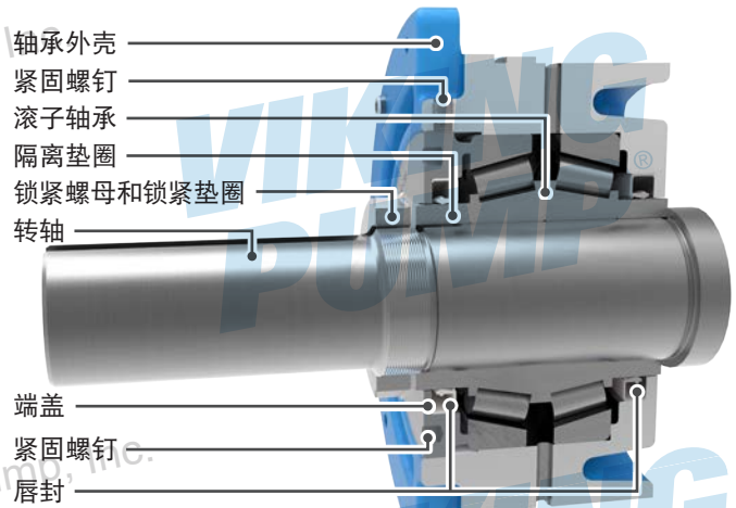
图 11: 轴承外壳组件 (Q、QS)
