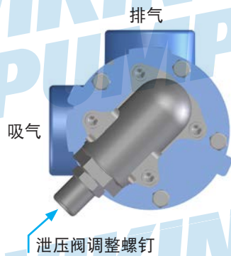
图 6: 泄压阀位置
