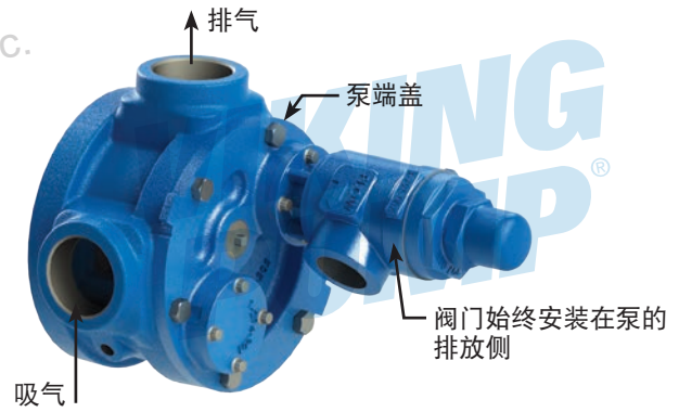
图 A5-B: 返罐式泄压阀
