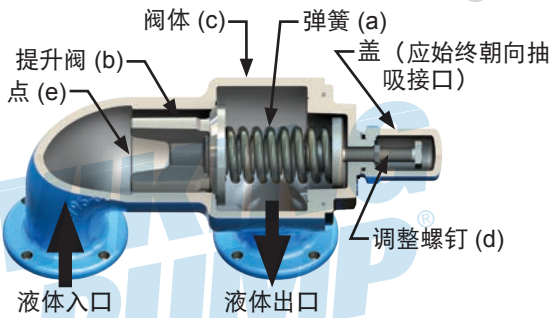
图 A4: 威肯内部 泄压阀的剖视图
