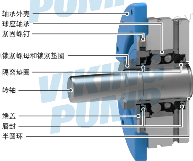
图 10: 轴承外壳组件 (K、KK、LQ、LL、LS)
