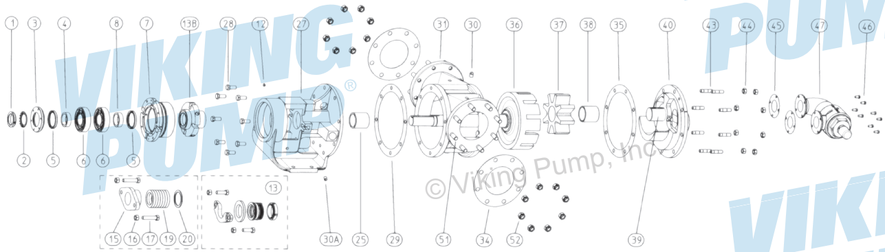
图 5: 分解图 (Q、QS 尺寸) — 126A SERIES™、4126A SERIES™、226A SERIES™、4226A SERIES™ 注: 图像仅具有代表性
