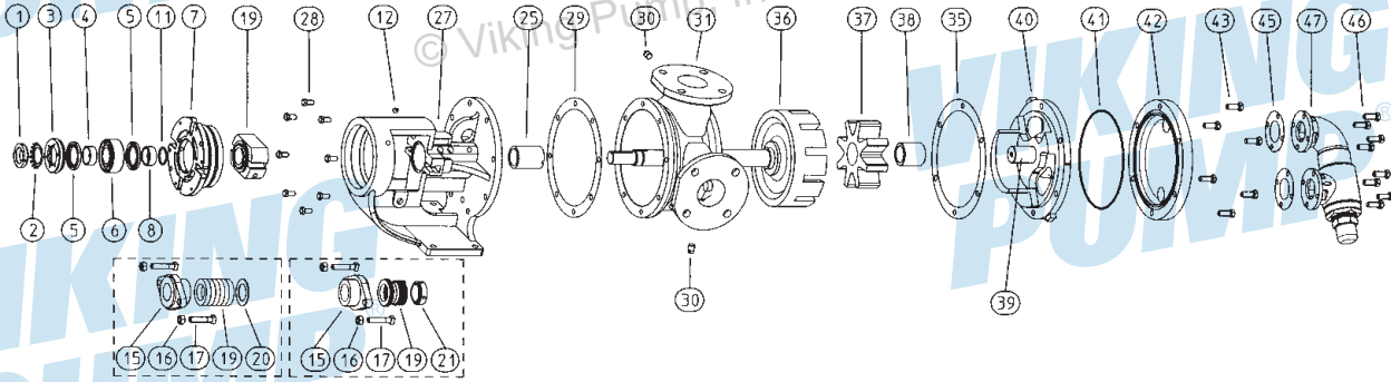
图 4: 分解图 (H、HL、K、KK、L、LQ、LL、LS 尺寸) — 126A SERIES™、4126A SERIES™、226A SERIES™、4226A SERIES™ 注: 图像仅具有代表性
