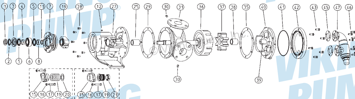
RAJAH 6: PANDANGAN TERBURAI (SAIZ H, HL, K, KK, LQ, LL, LS) — 127A SERIES™, 4127A SERIES™, 227A SERIES™, 4227A SERIES™ NOTA: IMEJ ADALAH WAKIL SAHAJA
