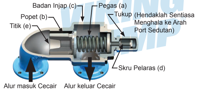
RAJAH A5-A: INJAP PELEGA TEKANAN DALAMAN
