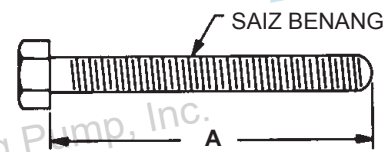
RAJAH 11: PANJANG MINIMUM SKRU BICU
