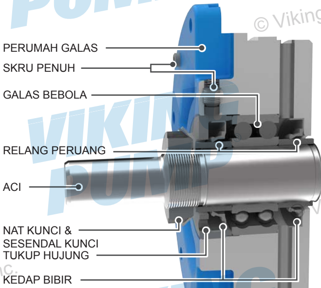
RAJAH 12: PEMASANGAN PERUMAH GALAS (H, HL)
