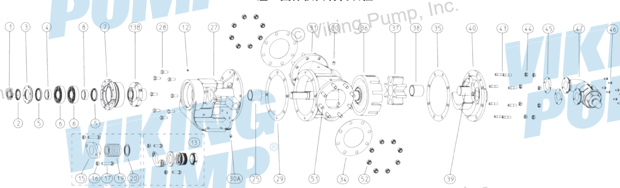
图 7: 分解图 (Q、QS 尺寸) — 127A SERIES™、4127A SERIES™、227A SERIES™、4227A SERIES™ 注: 图像仅具有代表性
