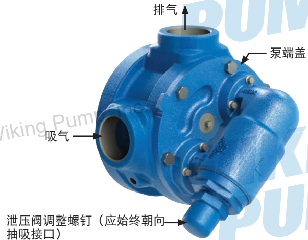
图 A5-A: 内部泄压阀
