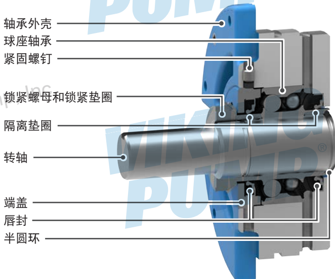
图 13：轴承外壳组件（K、KK、LQ、LL、LS）
