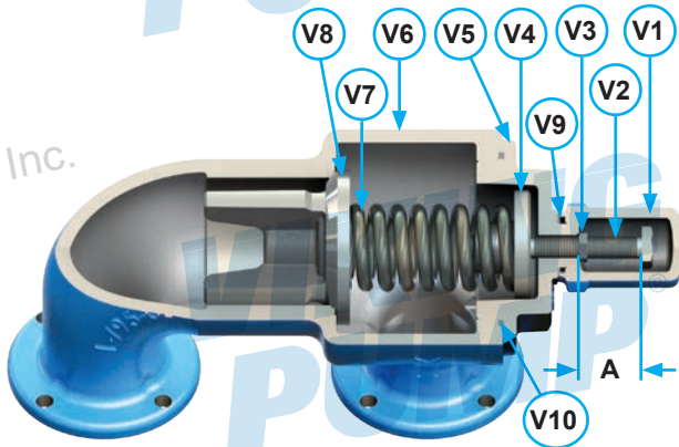
阀 - 零件列表
