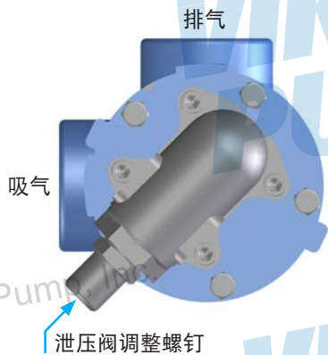
图 5：泄压阀位置
