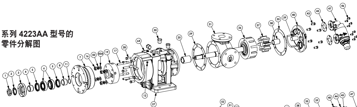
系列 4323AA 型号的 零件分解图
