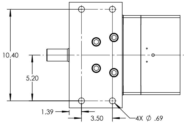
VIEW A-A
