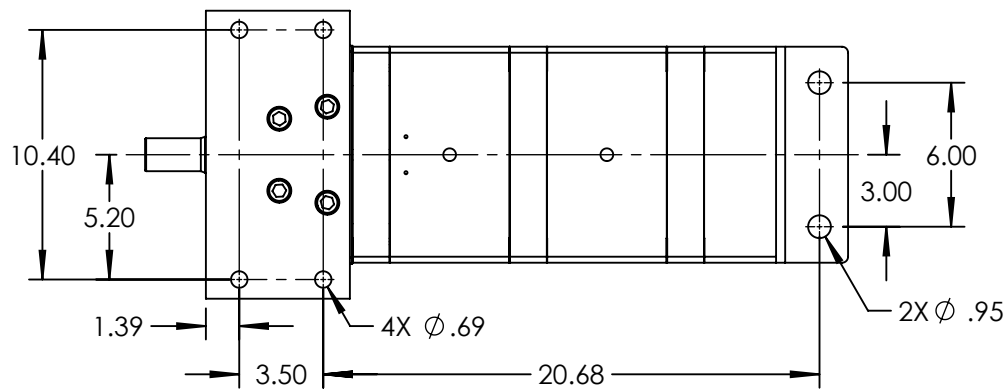
VIEW A-A
