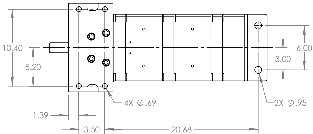
VIEW A-A
