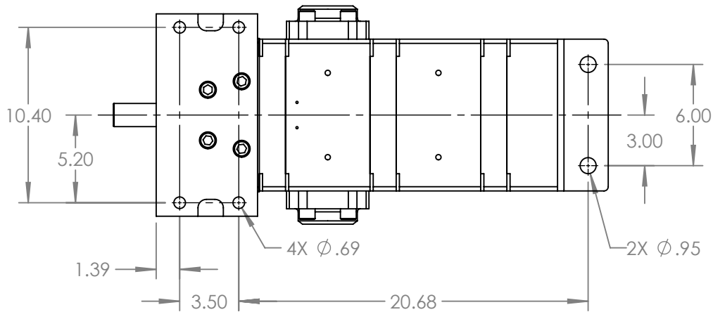
VIEW A-A
