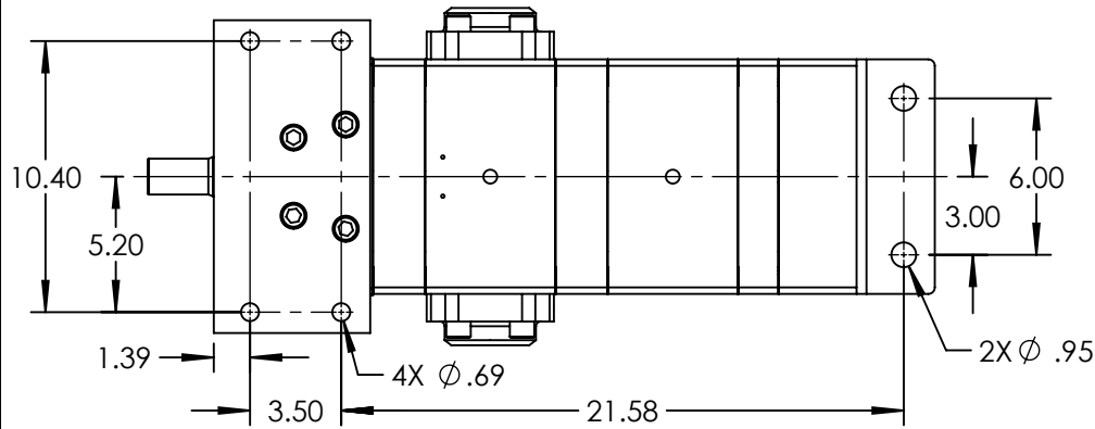
VIEW A-A
