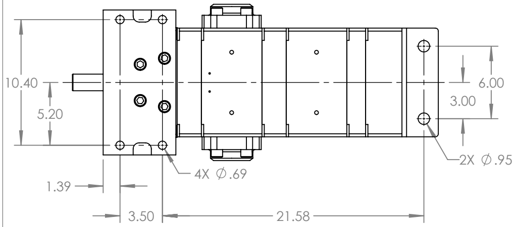
VIEW A-A
