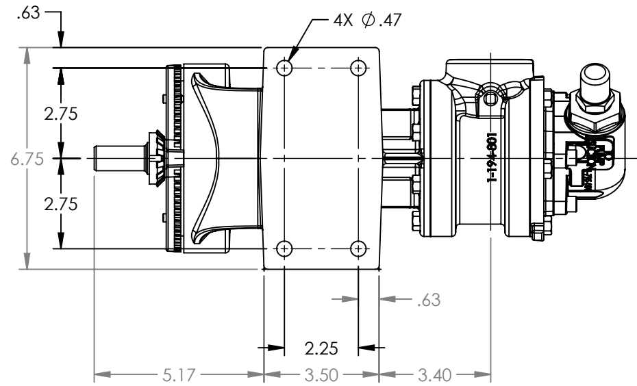
VIEW A-A
