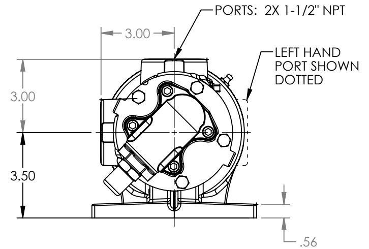
VIEW A-A
