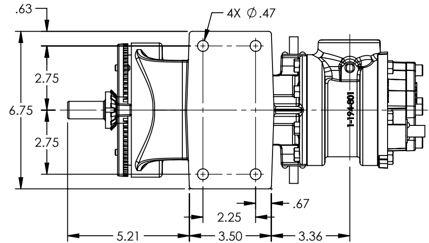
VIEW A-A
