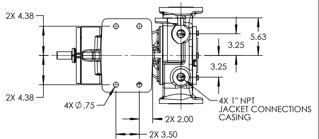
VIEW A-A
