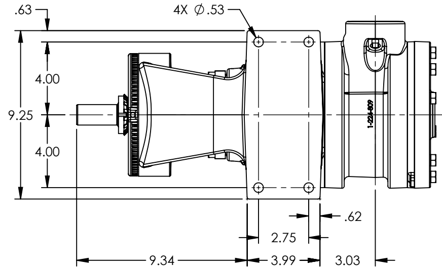
VIEW A-A
