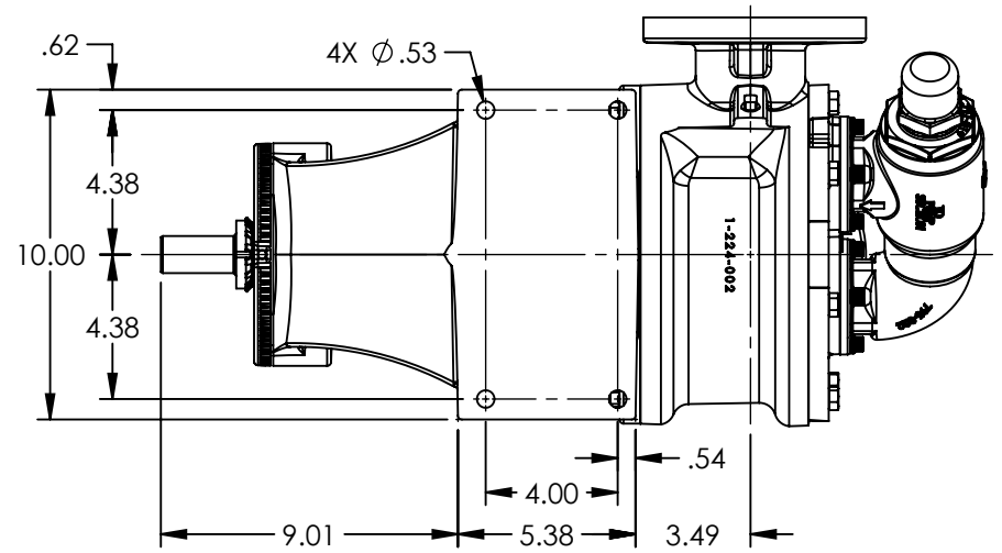
VIEW A-A
