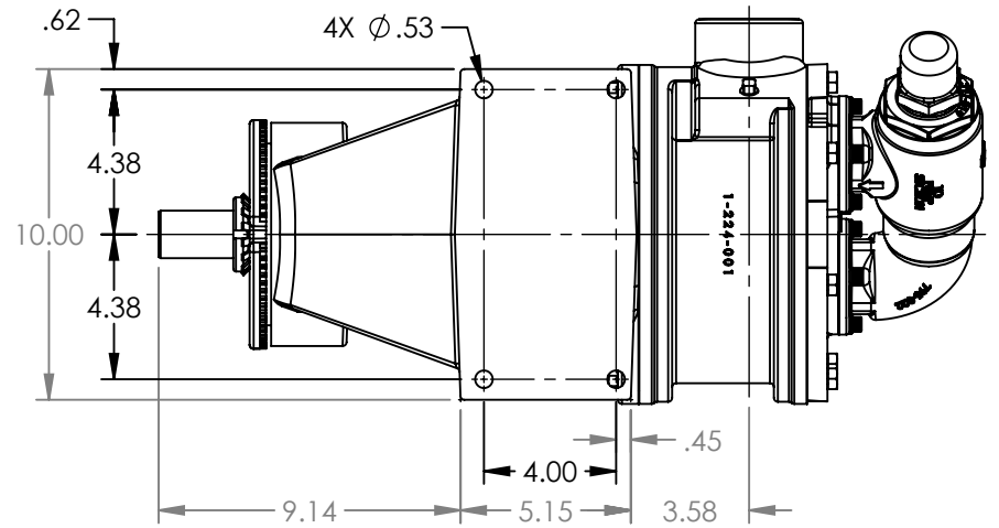
VIEW A-A
