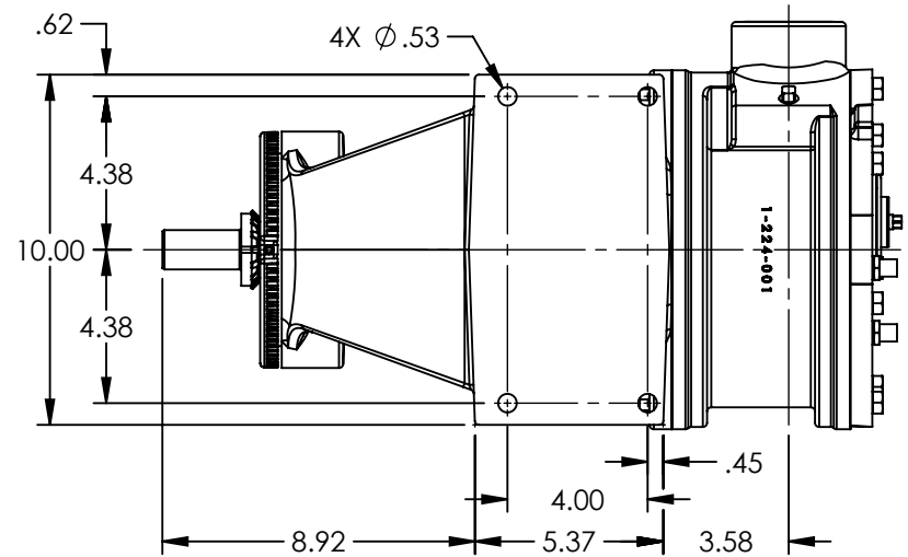
VIEW A-A
