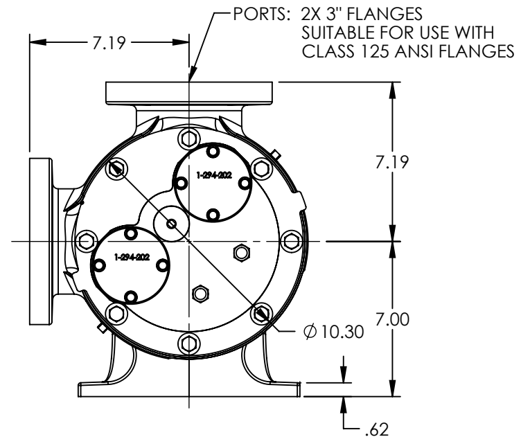
VIEW A-A
