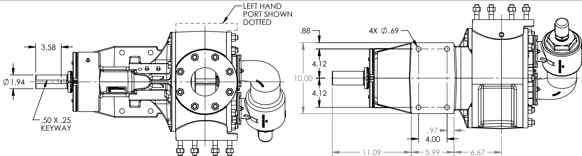
VIEW A-A
