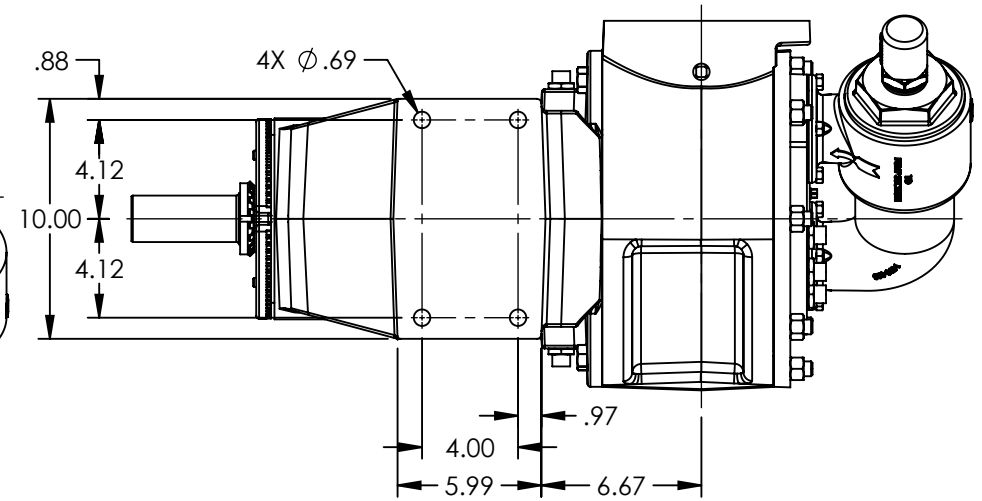
VIEW A-A
