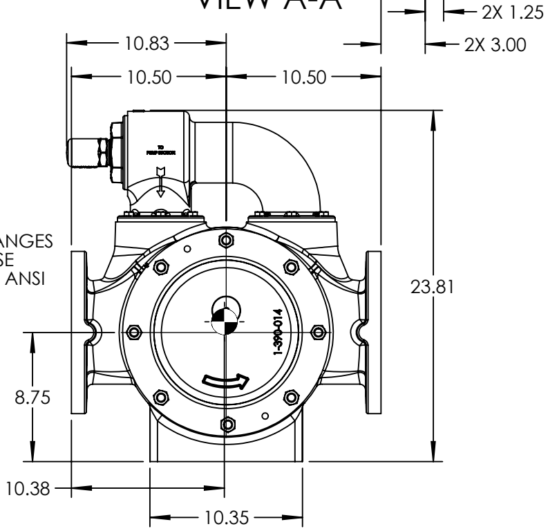
VIEW A-A
