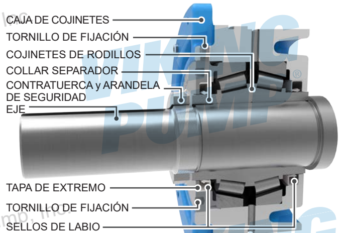
FIGURA 11: MONTAJE DE LA CAJA DE COJINETES (Q, QS)
