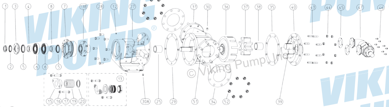
FIGURA 5: VISTA DESPIEZADA (TAMAÑOS Q, QS) — 126A SERIES™, 4126A SERIES™, 226A SERIES™, 4226A SERIES™ NOTA: LA IMAGEN ES SOLO REPRESENTATIVA.
