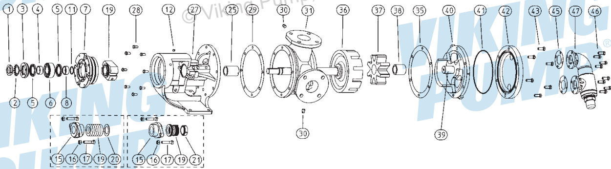
FIGURA 4: VISTA DESPIEZADA (TAMAÑOS H, HL, K, KK, L, LQ, LL Y LS) — 126A SERIES™, 4126A SERIES™, 226A SERIES™, 4226A SERIES™ NOTA: LA IMAGEN ES SOLO REPRESENTATIVA.
