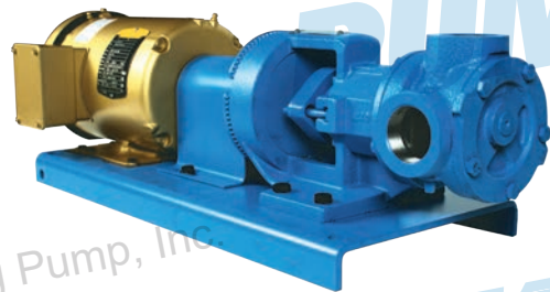
FIGURA A11: TRANSMISIÓN DIRECTA
