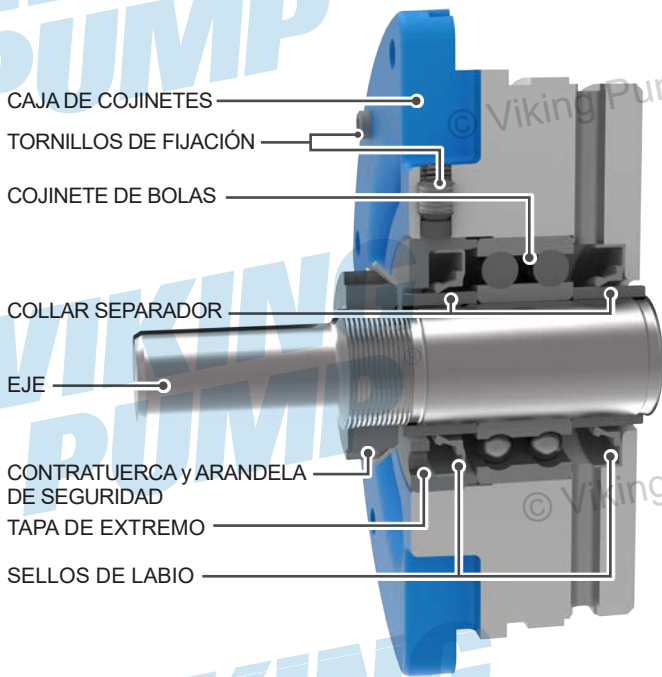
FIGURA 9: MONTAJE DE LA CAJA DE COJINETES (H, HL)
