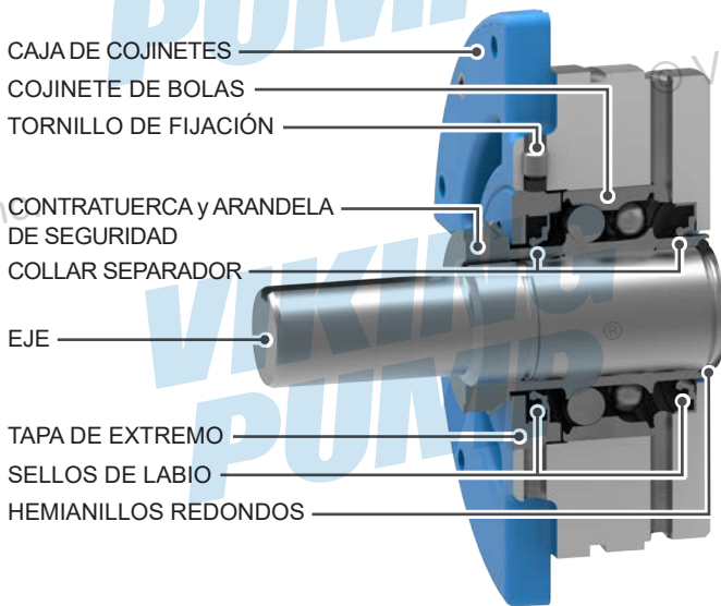
FIGURA 10: MONTAJE DE LA CAJA DE COJINETES (K, KK, L, LQ, LL Y LS)
