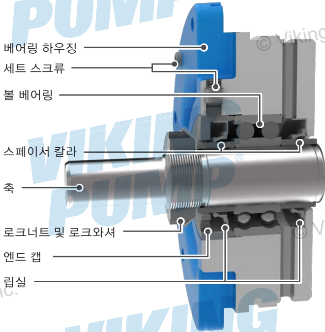
그림 12: 베어링 하우징 조립체(H, HL)
