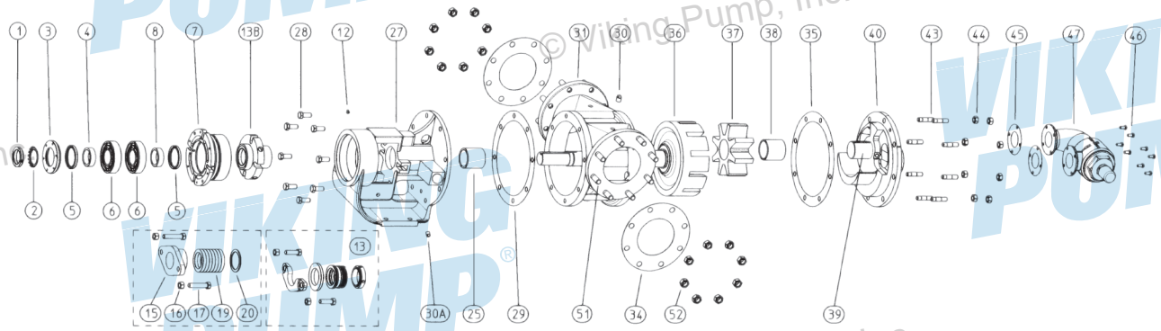
그림 7: 분해도(Q, QS 크기) — 127A SERIES™, 4127A SERIES™, 227A SERIES™, 4227A SERIES™ 주의사항: 참조용 이미지입니다.
