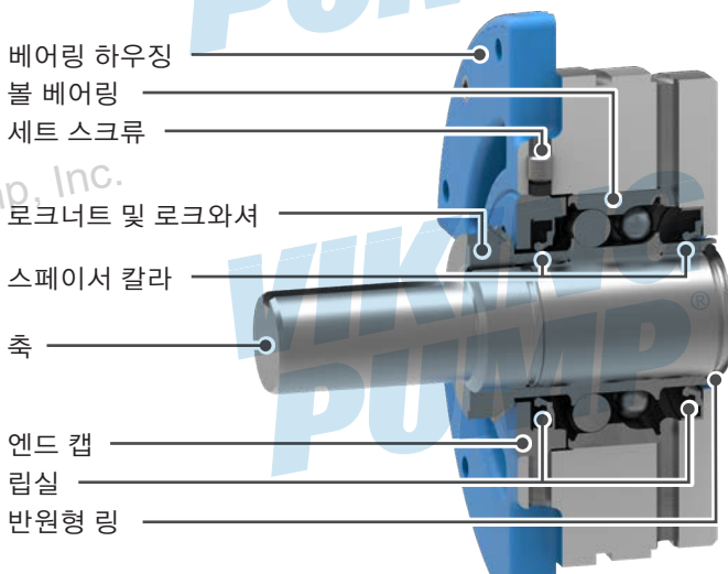
그림 13: 베어링 하우징 조립체 (K, KK, LQ, LL, LS)
