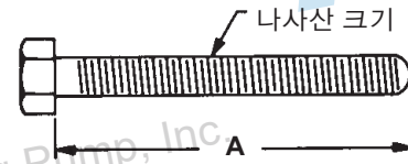
그림 11: 잭스크류의 최소 길이
