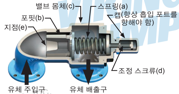
그림 A4: VIKING 내부 압력 배출 밸브 도해
