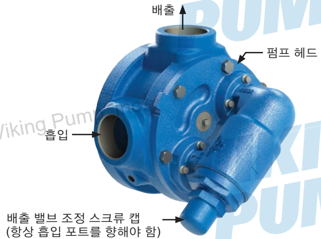
그림 A5-A: 내부 압력 배출 밸브
