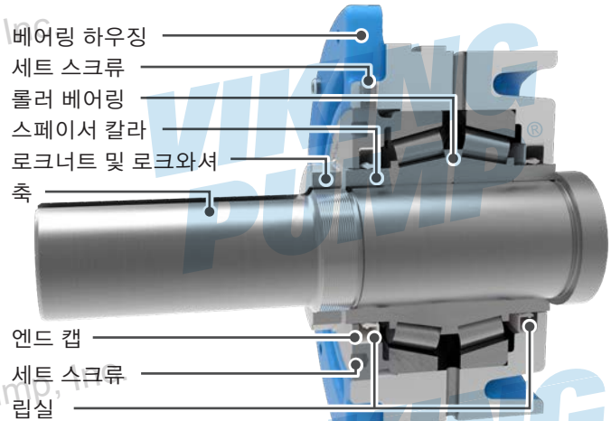
그림 14: 베어링 하우징 조립체 (Q, QS, N, R, RS)
