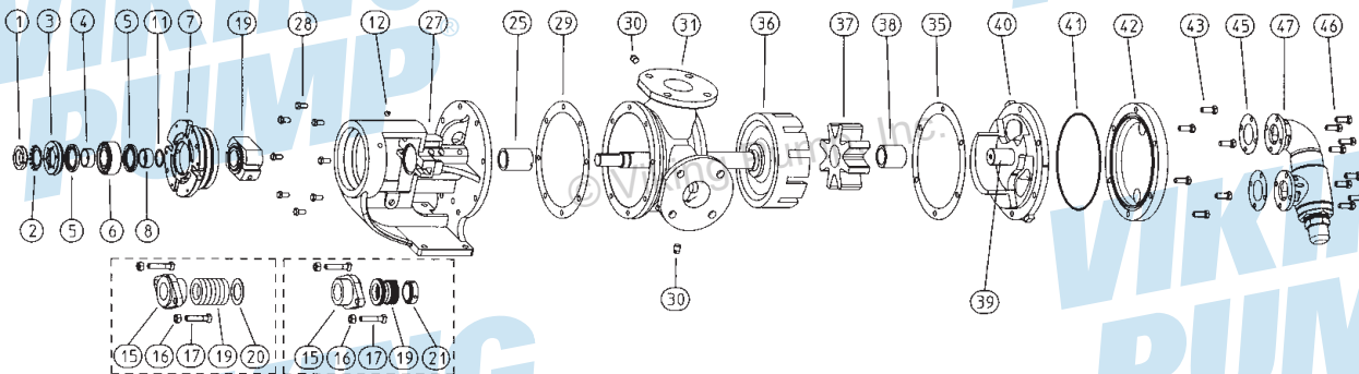
그림 6: 분해도(H, HL, K, KK, LQ, LL, LS 크기) — 127A SERIES™, 4127A SERIES™, 227A SERIES™, 4227A SERIES™ 주의사항: 참조용 이미지입니다.
